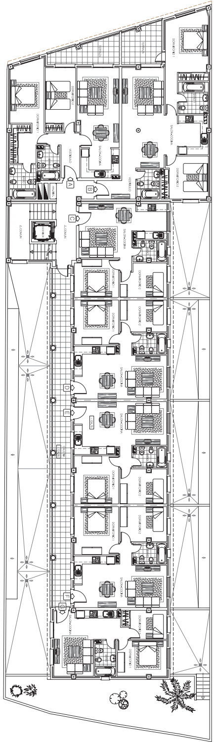
PLANTA ALTA - NIVEL +104.76
